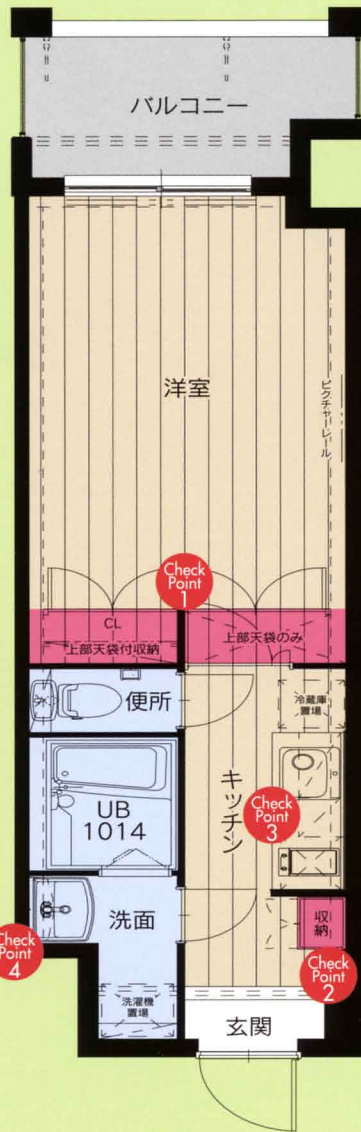
B1 1K TYPE 専有面積 27.86㎡
